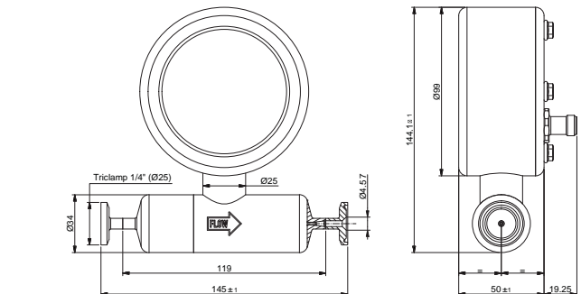
Соединение с трубопроводом фланцевого типа (Triclamp)
